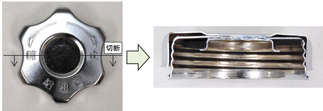
写真4. 漏えいが確認されたキャップの断面
